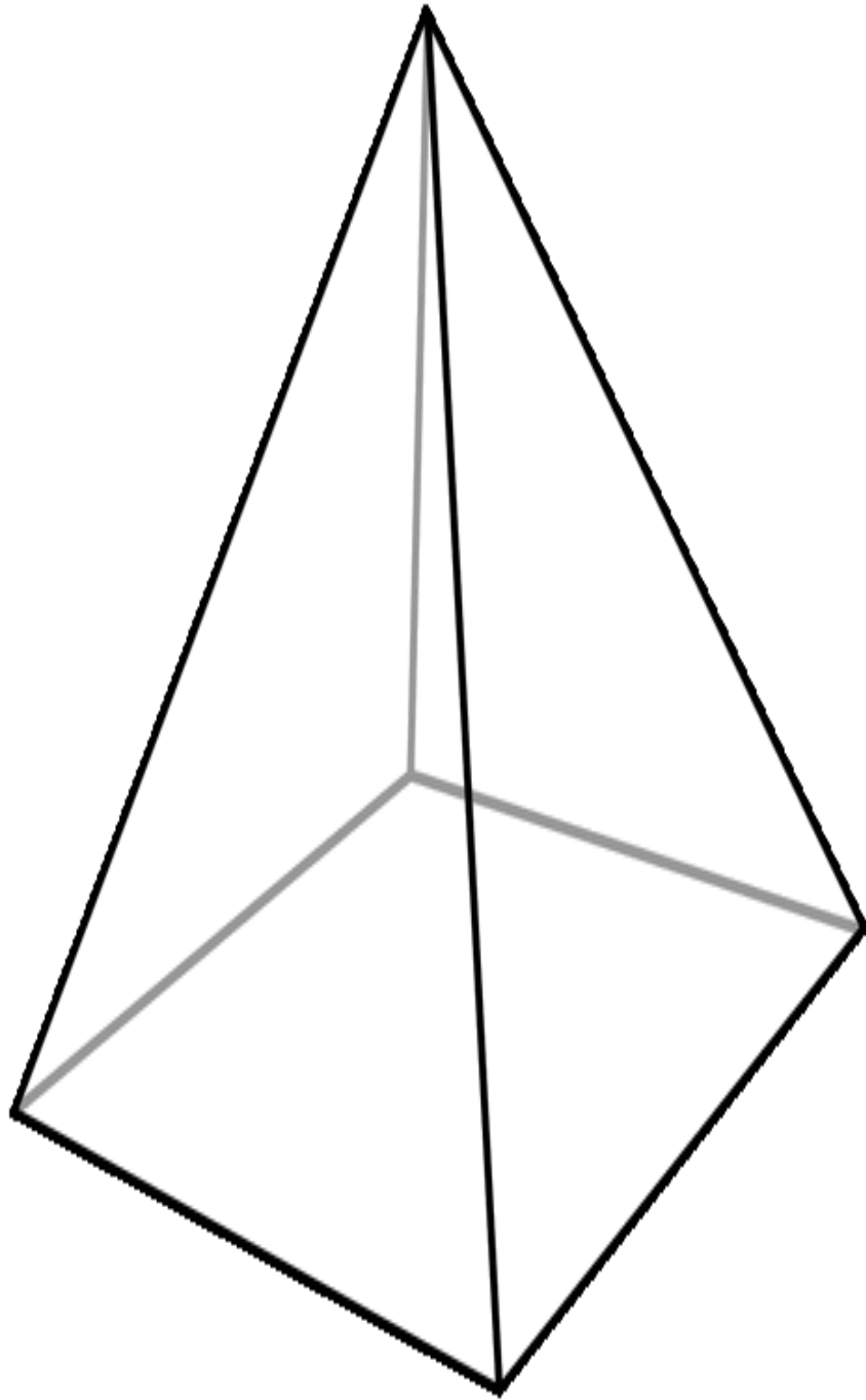
棱锥体
