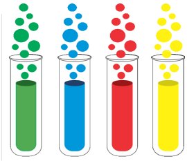
试管
