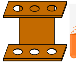
试管架
